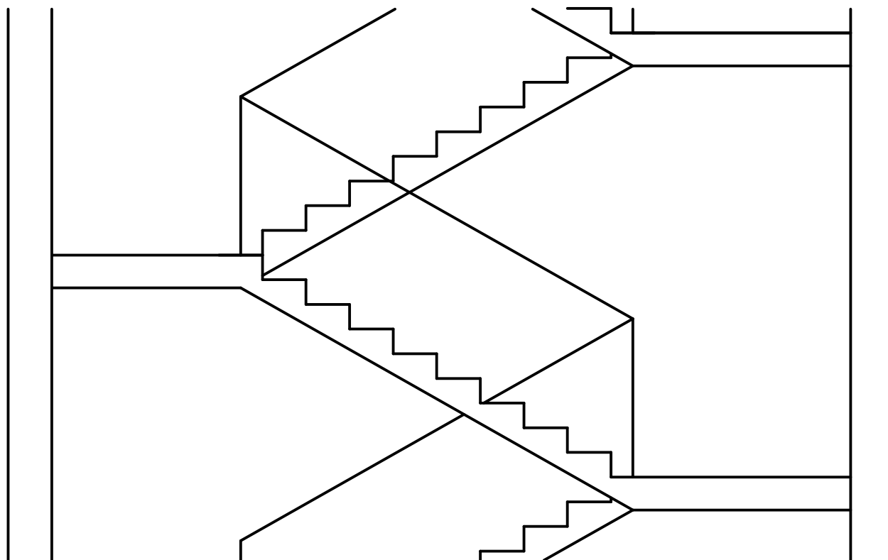
HOSSZMETSZET
