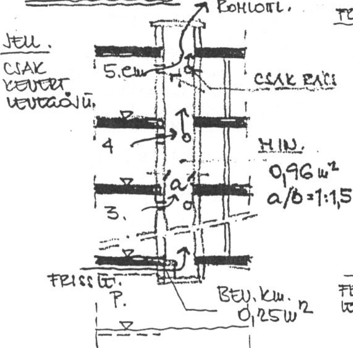
Egyaknas metszete
