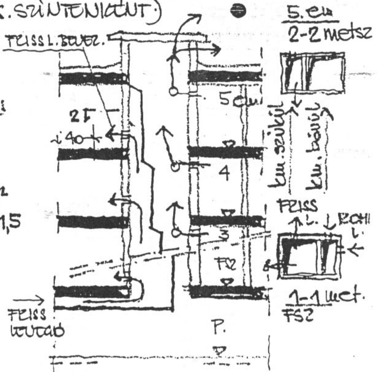
Kétaknas tvi metszete
