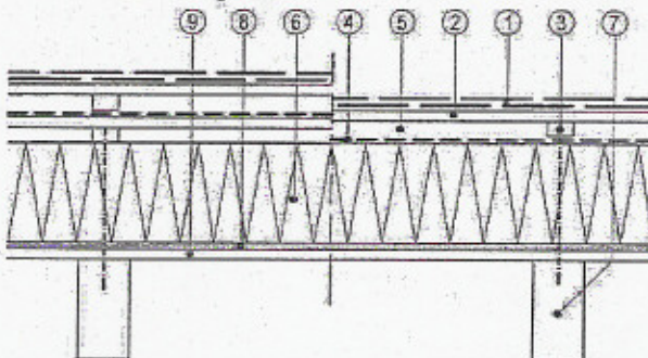
a, Kétszeresen átszellőztetett tetőszerkezet
