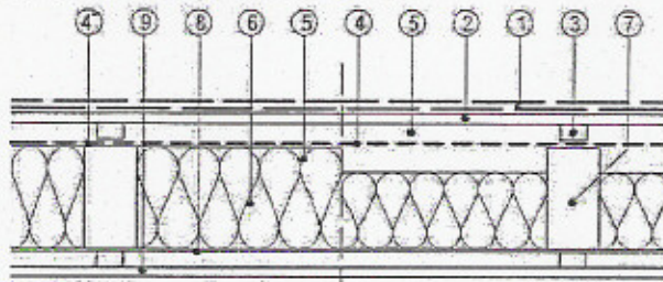
a, Kétszeresen átszellőztetett tetőszerkezet
