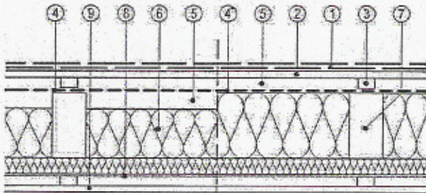
a, Kétszeresen átszellőztetett tetőszerkezet
