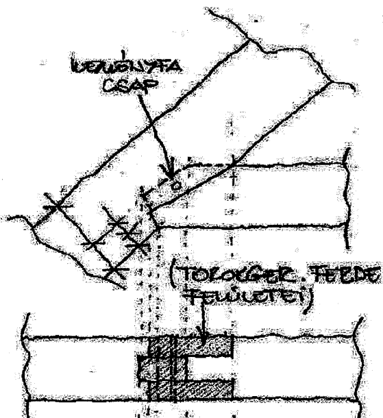
FELES CSAPOS BEÉPESÍTÉS
