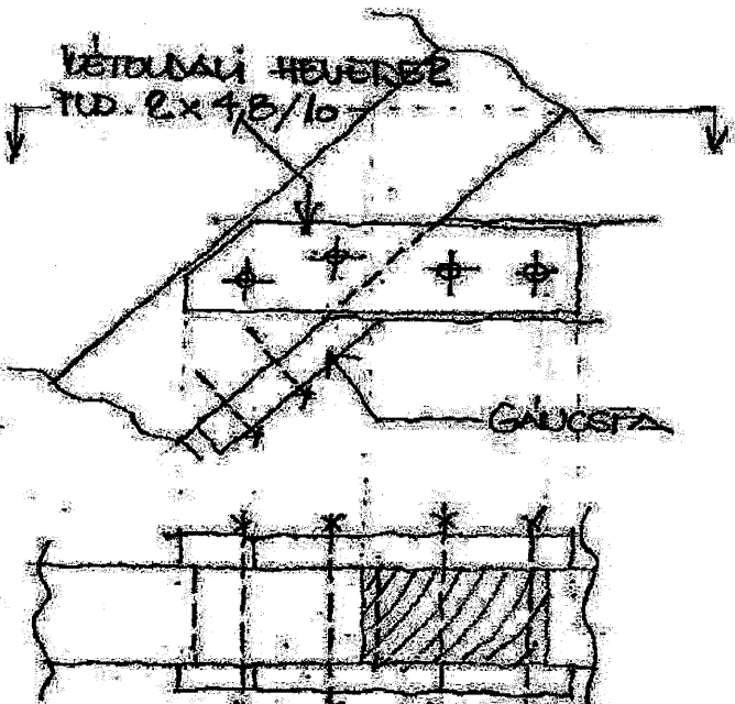
FELES CSAPOS BEÉPESÍTÉS
