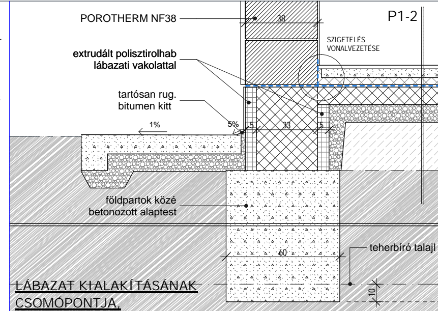
Metszetek
