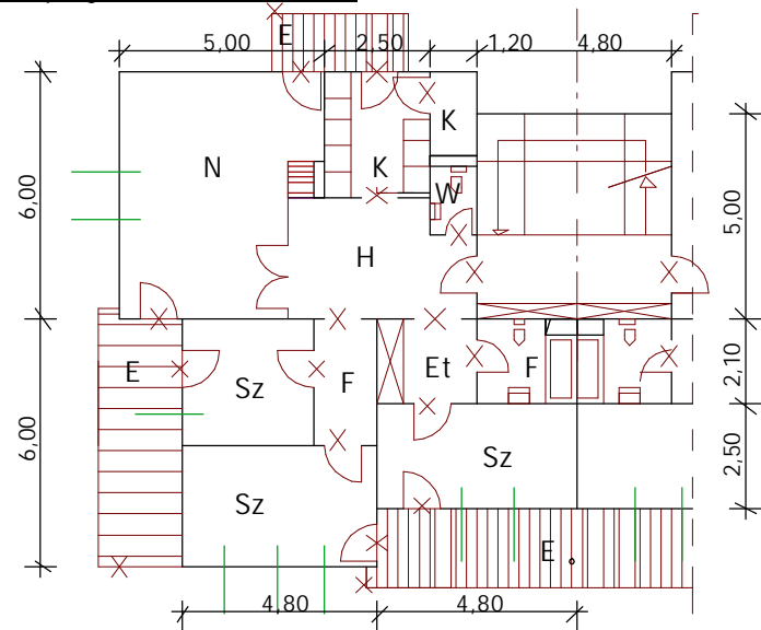
Alaprajz
