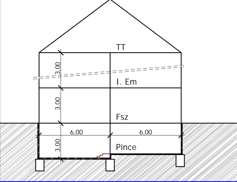
Metszet vázlat M=1:200
