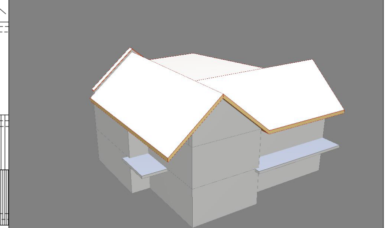
Nyeregtető beforduló gerinccel nyaktaggal, lapos hailás-szögű tetővel kiegészítve
