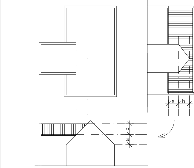
Összemetszések eltérő magasságú párkányok esetén
