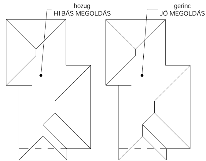
Összemetsződés szerkesztési sémája
