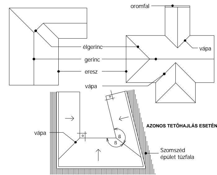
Tetőidom szerkesztés szabályai
