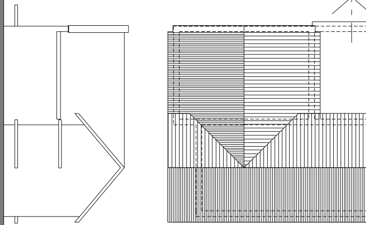
Nyeregtető hosszirányú gerinccel és "L" alakban beforduló nyereg-fiók tetővel
