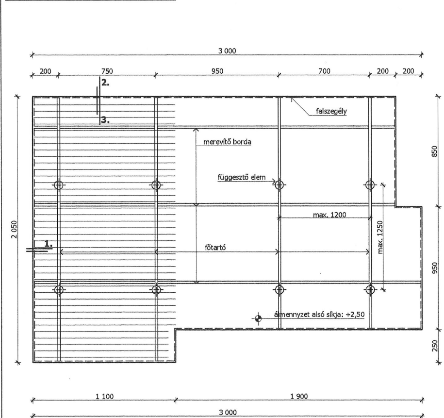
Sávos fém álmennyezet terve M=1:20
