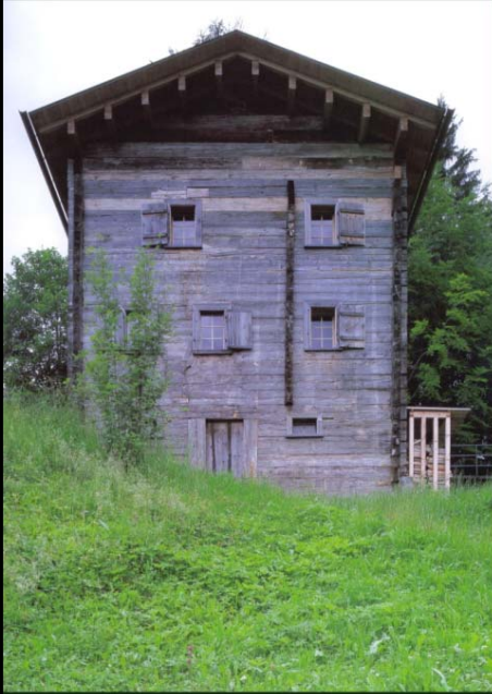
Peter Zumthor: Gugalun ház, Versam, Svájc, 1990-1994
