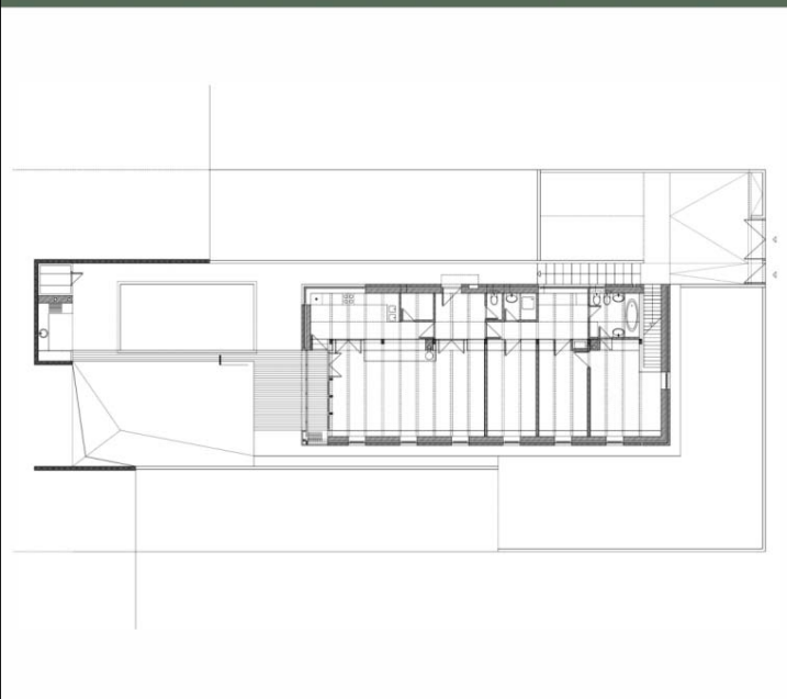
Balázs Mihály: Családi ház, Tinnye, 2002
