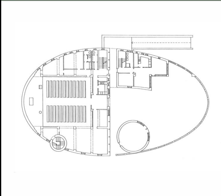
Nagy Tamás: Evangélikus templom és parókia, Dunaújváros, 1996
