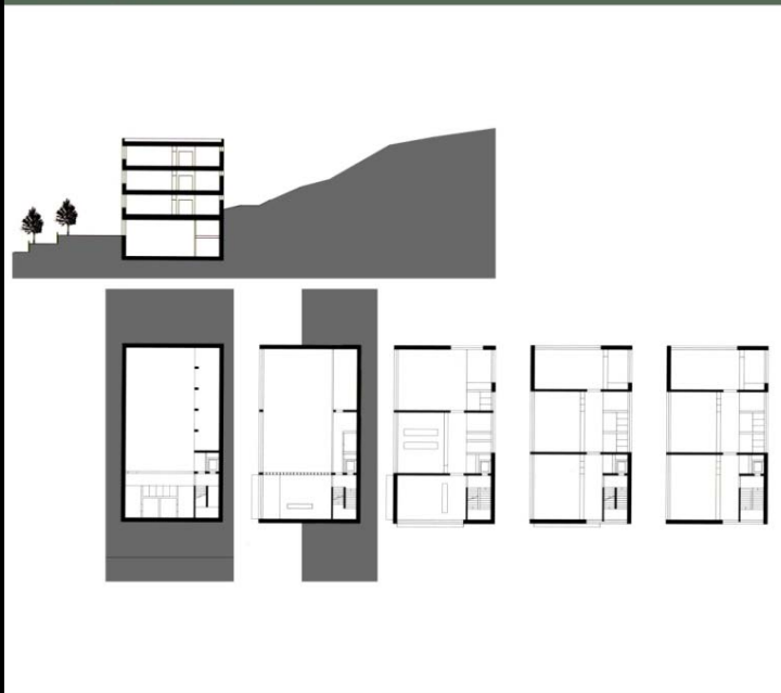
cukrowicz.nachbaur architekten (Andreas Cukrowicz): Általános iskola és óvoda, Doren, 2003
