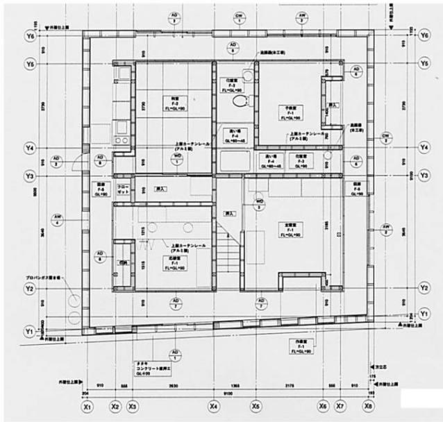
Kazuyo Sejima Ryue Nishizawa: S-ház, Okayama, Japán, 1997
