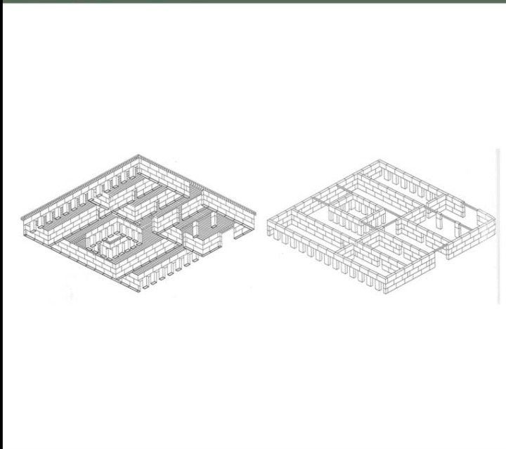
Gilles Perraudin, Françoise Jourda: Borraktár, Vauvert, Franciaország
