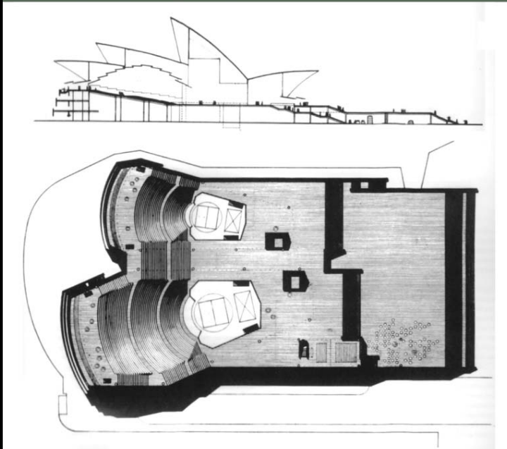
Jorn Utzon: Operaház, Sidney 1957-1973
