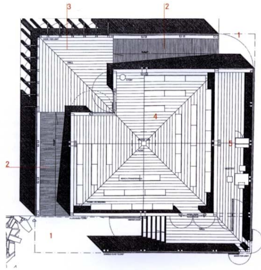
Ansi Lassila: Templom, Karsamaki, Finnország, 2004
