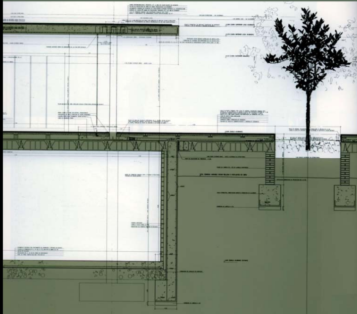
Alberto Campo Baeza: Innovatív technológiai központ, Mallorca, Spanyolország, 1998
