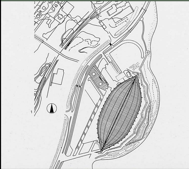
Niels Torp: Olimpiai jégcsarnok, Hamar, Norvégia, 1992
