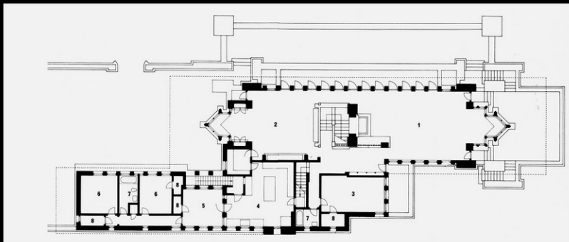
Robie-ház emeleti alaprajz
