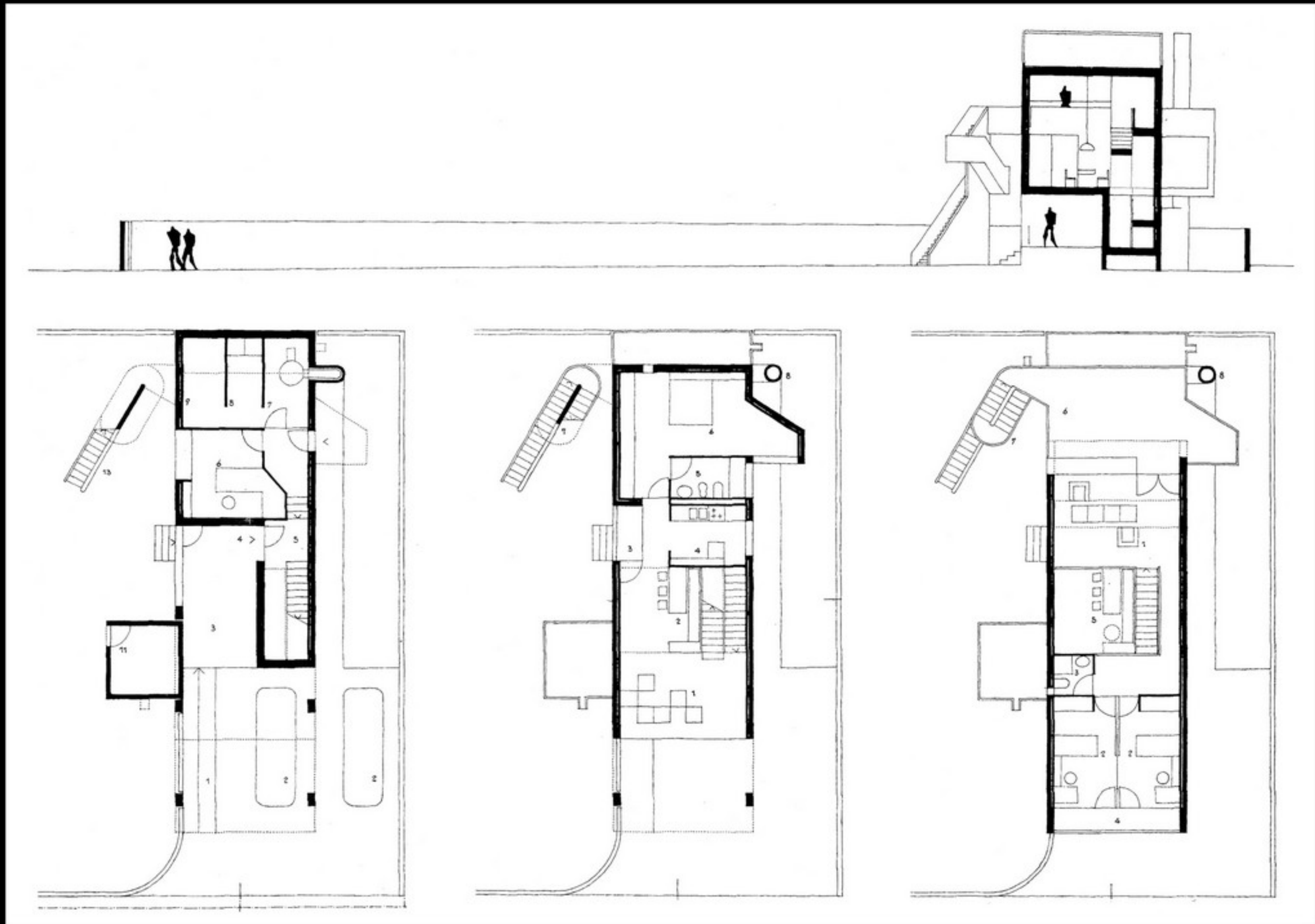
Stabio-i családi ház alaprajzai és metszete
