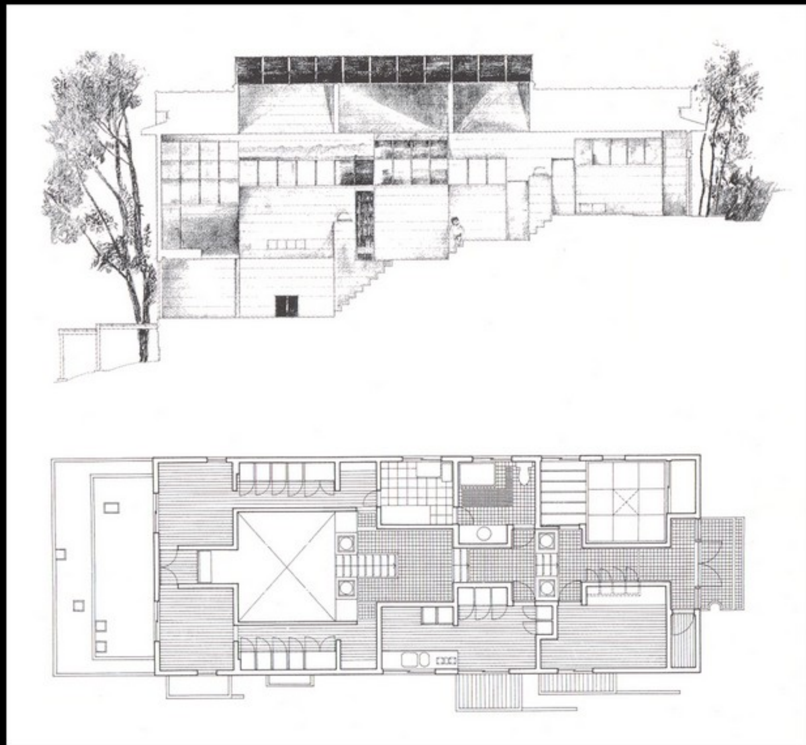
Hara-ház belső, alaprajz és metszet
