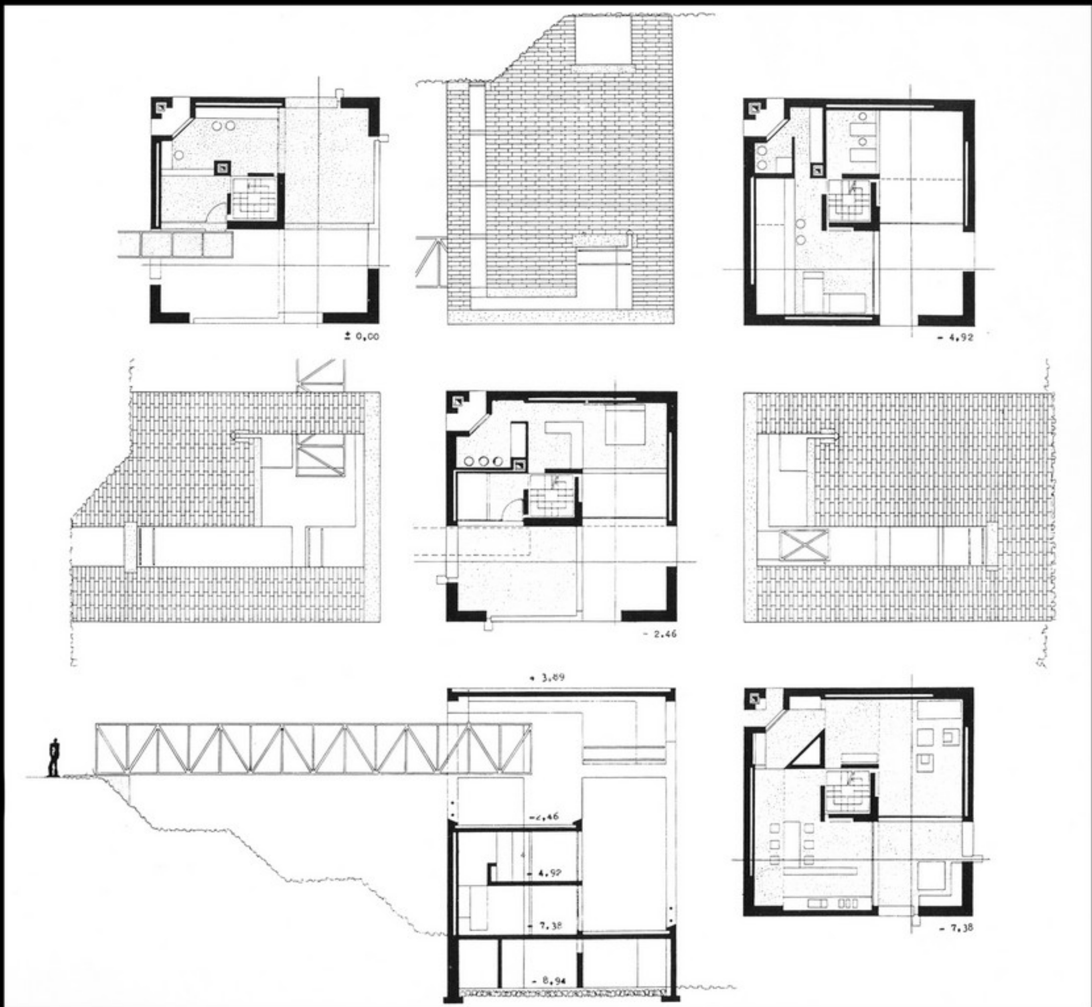
Bianchi-ház, alaprajzok, metszet, homlokzatok
