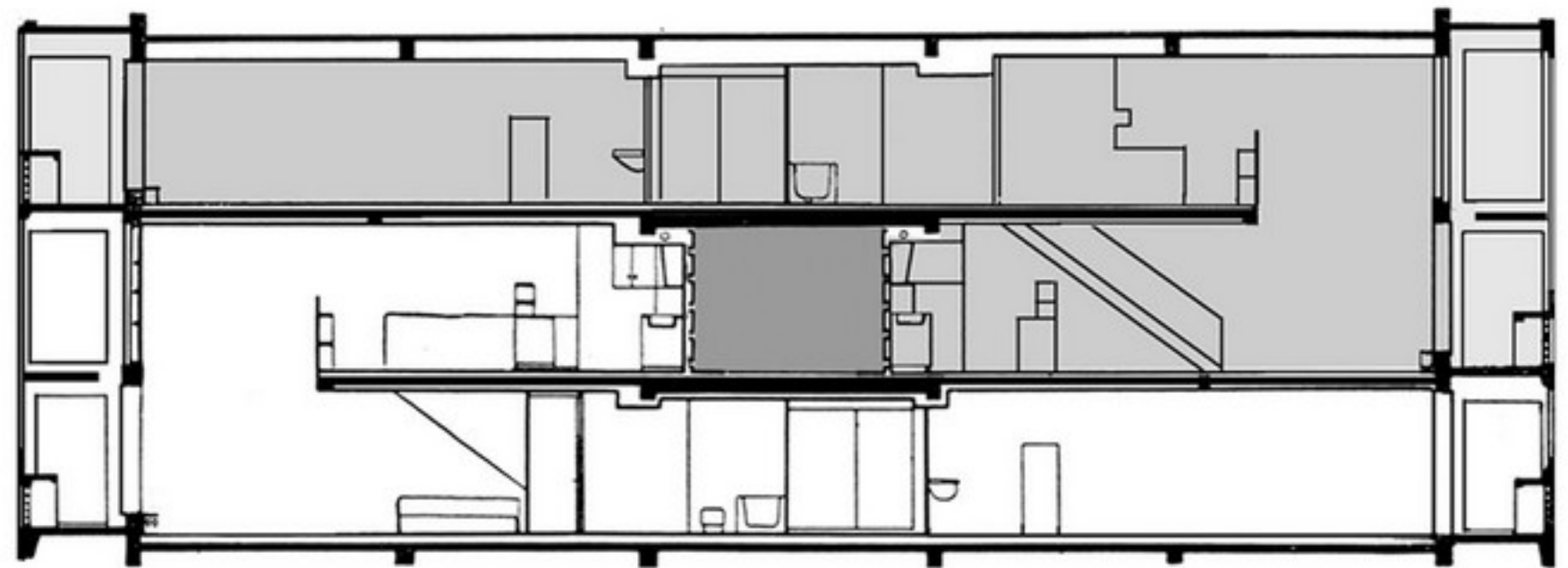
METSZET
