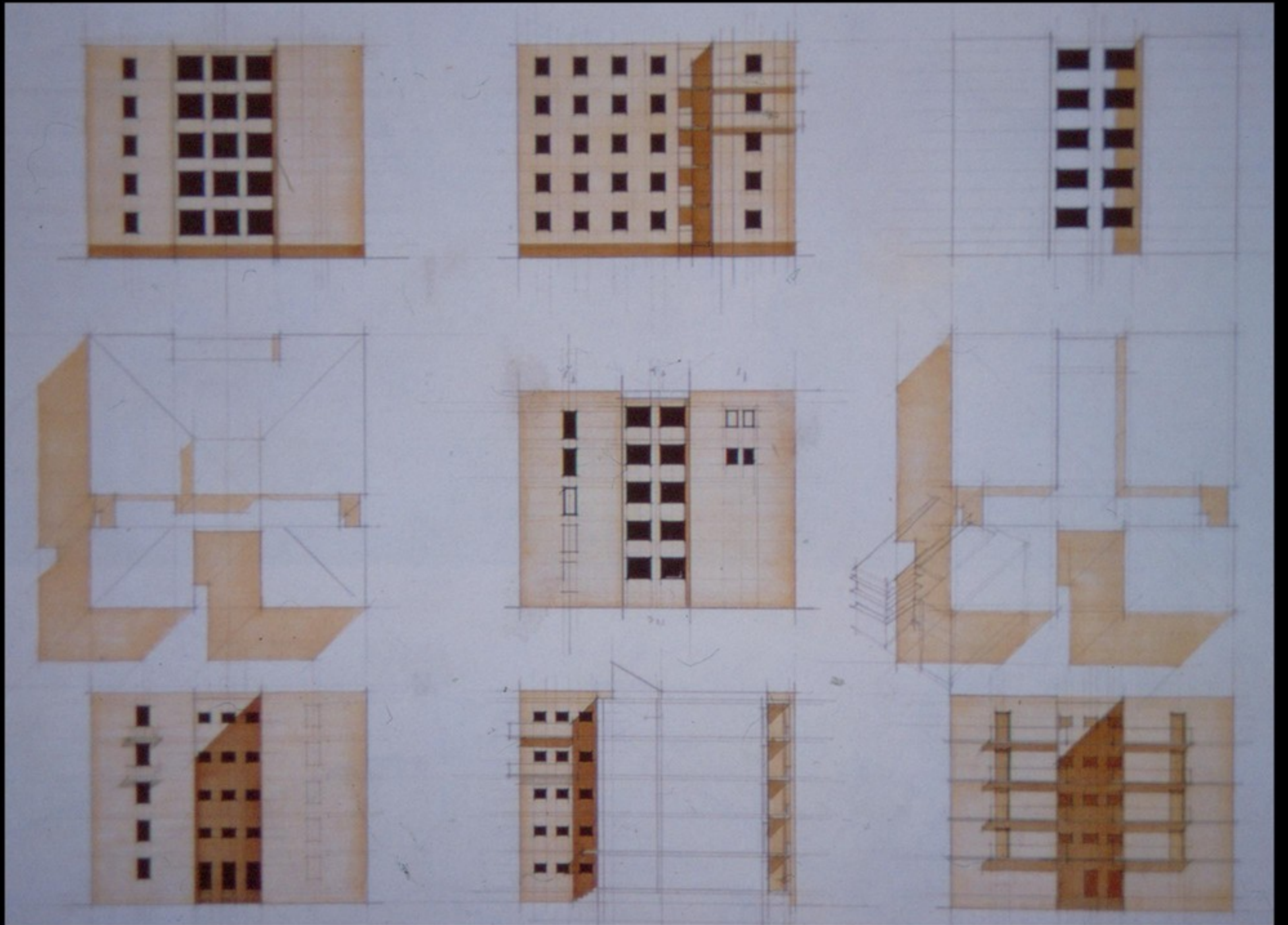
Berlin, Rauchstrasse - Aldo Rossi
