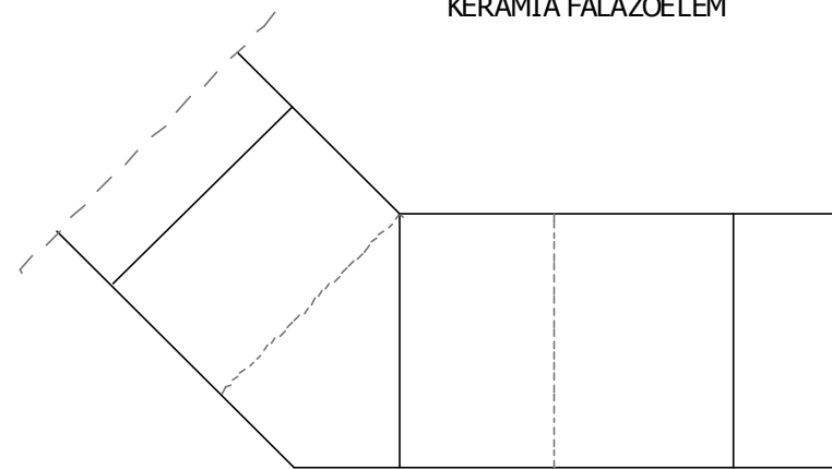
TOMPASZÖGŰ FALSAROK PÓRUSBETON FALAZÓELEM
