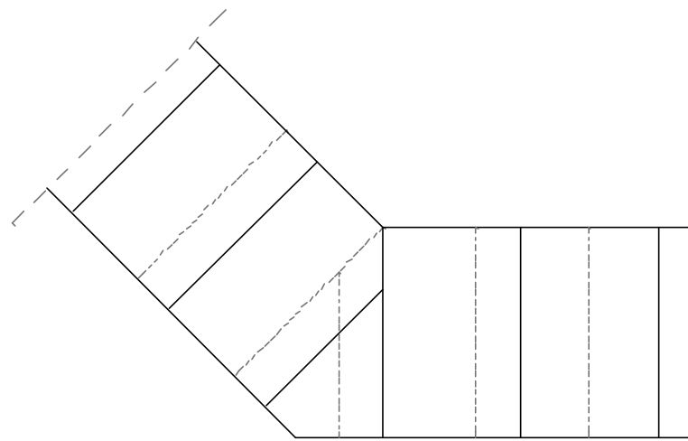
TOMPASZÖGŰ FALSAROK KERÁMIA FALAZÓELEM
