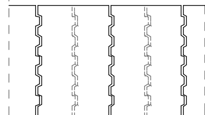
NÚTFÉDERES, ÜREGES KERÁMIA FALAZÓELEM
