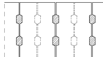
HABARCSTÁSKÁS, ÜREGES KERÁMIA FALAZÓELEM
